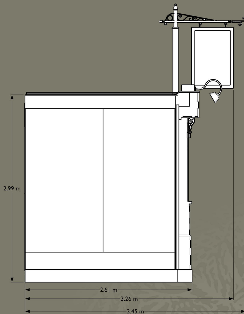
End Elevation
